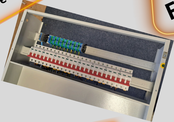
Vložka vystrojená
